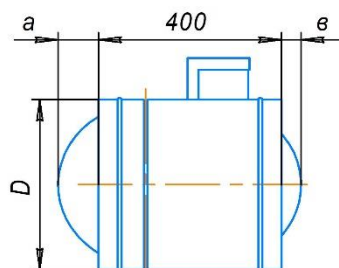
Рис.3. Размеры вылета заслонки в открытом положении за пределы клапана исполнений HO-AxB
